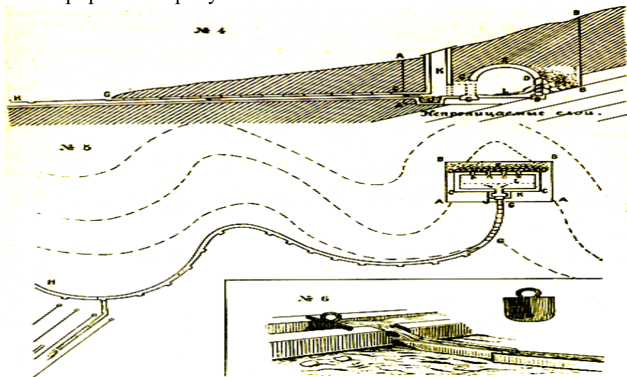
Рис. 3 – Схема водопровода для орошения виноградников
